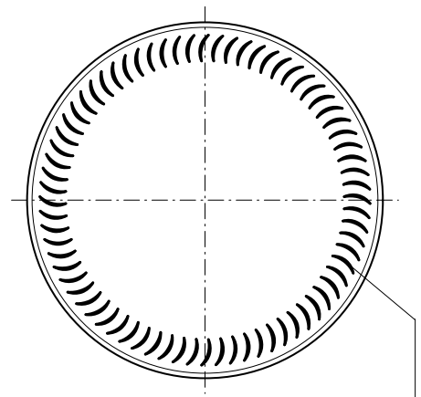
Standfläche geriffelt 72 Segmente h=0,5^{±0,1} mm tief
