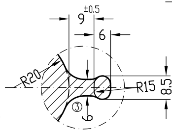
Schnitt D-D
